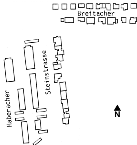
Individuell realisierte Einfamilienhausüberbauungen Haberacher, Steinstrasse und Breitacher. Dank vorgegebener „Spielregeln“ entsteht dennoch eine Gesamtüberbauung. Quelle: 1)
